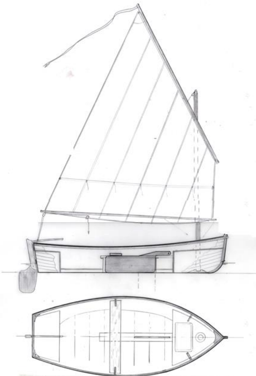
Algemeen Plan Zeilsloep Najork 13
